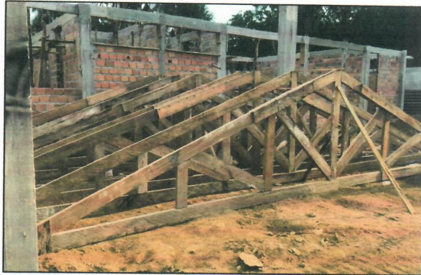
FOTO N° 07: CONFECCIÓN DE TIJERALES EN MODULO I Y PARA MODULO IV.
