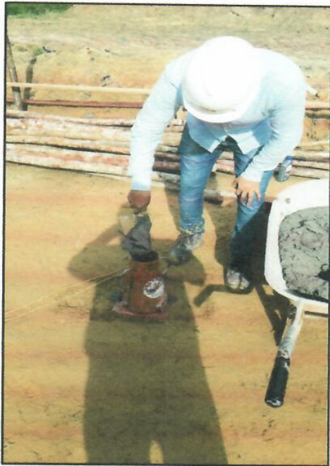
FOTO N°09: ENSAYO DE SLUMB EN MORTERO.
