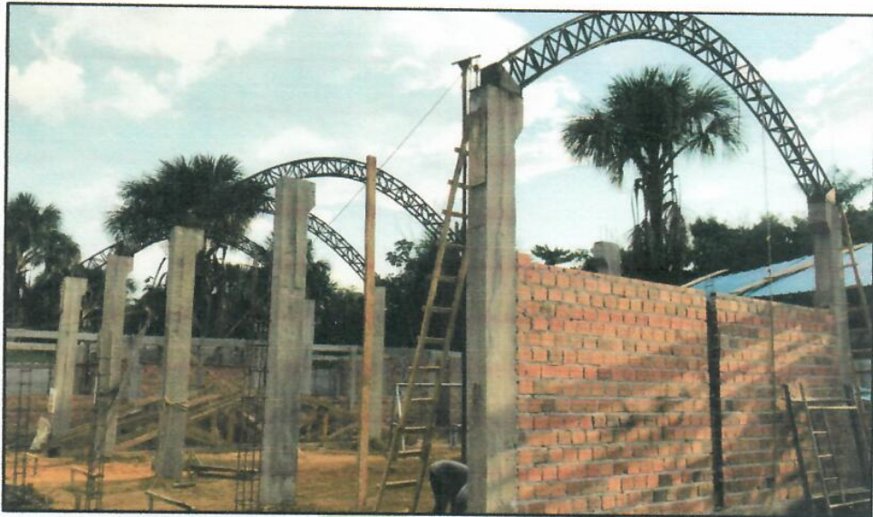
FOTO N°03: IZAJE DE TIJERALES METÁLICOS EN MODULO V.
